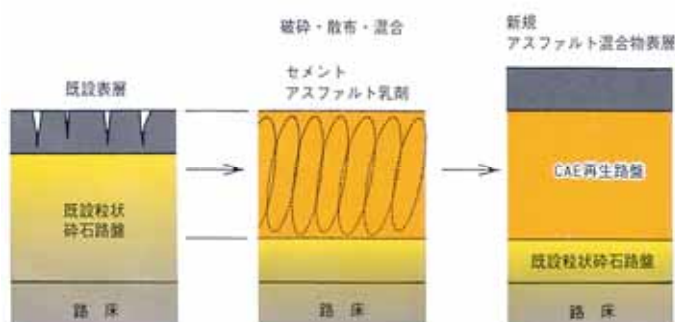
路上再生 CAE 路盤工法の概要
